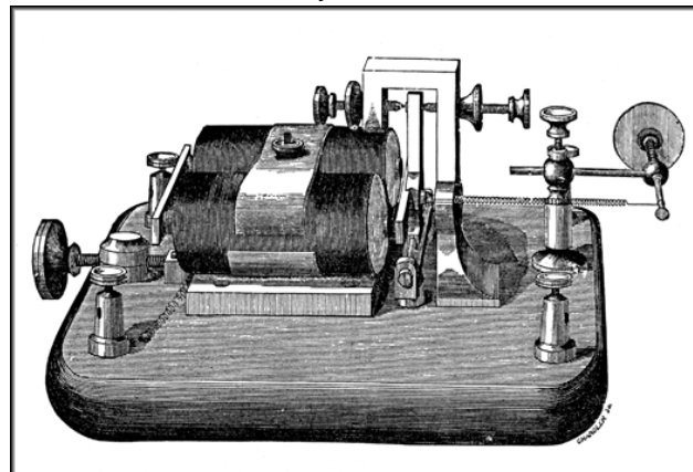
Morse-féle távíró készülék
