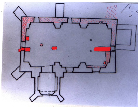
11. ábra A vörösberényi templom 1966-os feltáráskori alaprajza a legrégebbi falakkal
