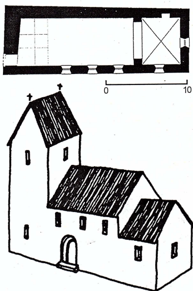
7. ábra A XI.-i templom alaprajza és elméleti rekonstrukciója
