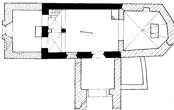
12. ábra Balatonfüred- temetői templomrom alapja
