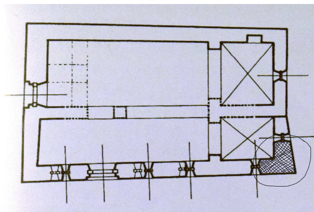
14. ábra A vörösbereányi református templom rekonstruált alaprajza 56
