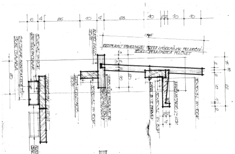
21. ábra Vörösberényi református templom B 4 padterve 165
